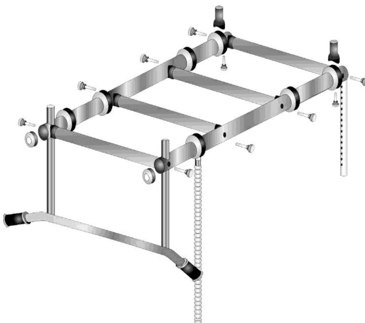
Рис.4 Установка распорных труб
